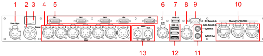
grandMA3 full-size CRV panneau arrière
