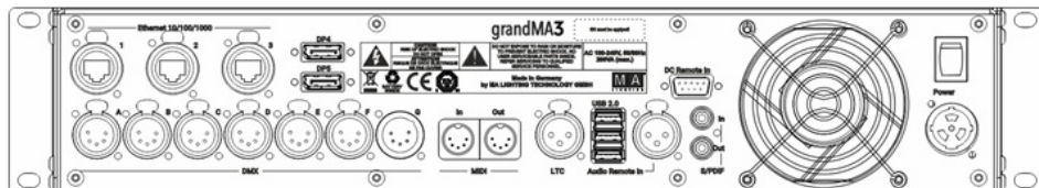
grandMA3 replay unit – panneau arrière
