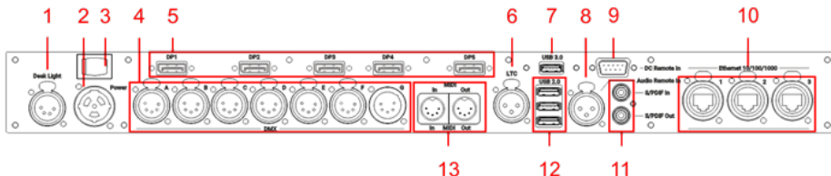
grandMA3 full-size CRV Rückseite
